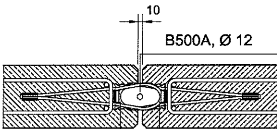
Bild 6: Minimale Fuge
