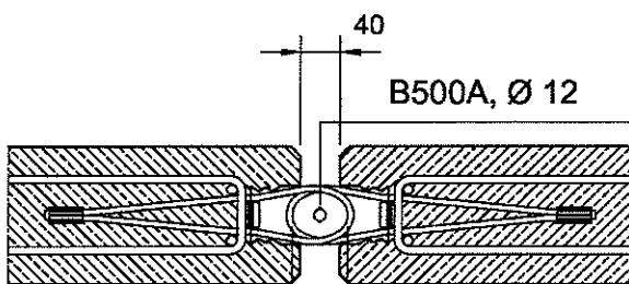
Bild 7: Maximale Fuge
