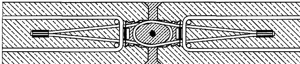
Bild 10: Wand - Wandverbindung
