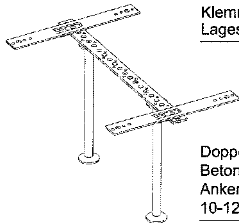
HDB-G-S - 2er Element
