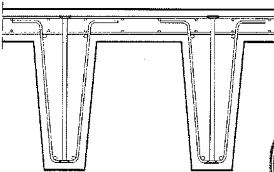
Beispiel 3: TT-Platte
