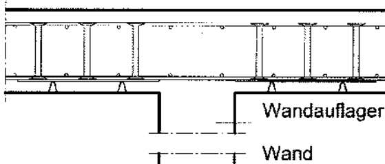
Beispiel 1: Platte
