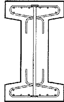
Beispiel 5: I- Träger
