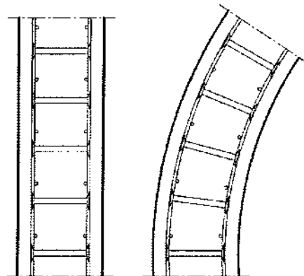
Beispiel 8: vertikale Plattenbauteile, Wand gerade, Wand gekrümmt
