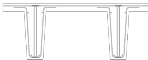
Beispiel 3: TT-Platte
