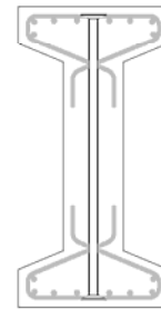
Beispiel 5: I-Träger
